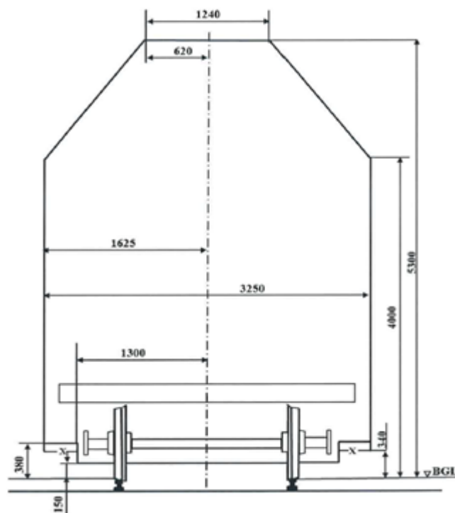
2 paveikslas. Pakrovos gabaritas 1 520 mm vėžės geležinkeliuose
