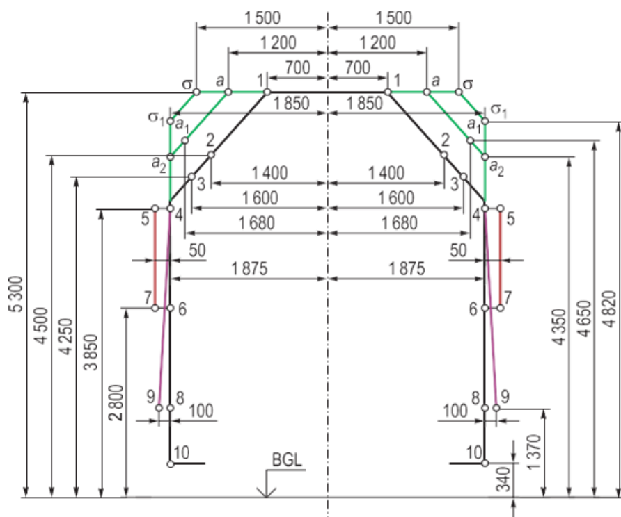
Geležinkelių riedmenų gabaritas T
