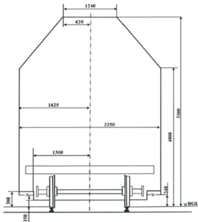
Pakrovos gabaritas 1520 mm vėžės geležinkeliuose
